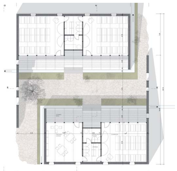
Grundriss des ausgewählten Entwurfs
